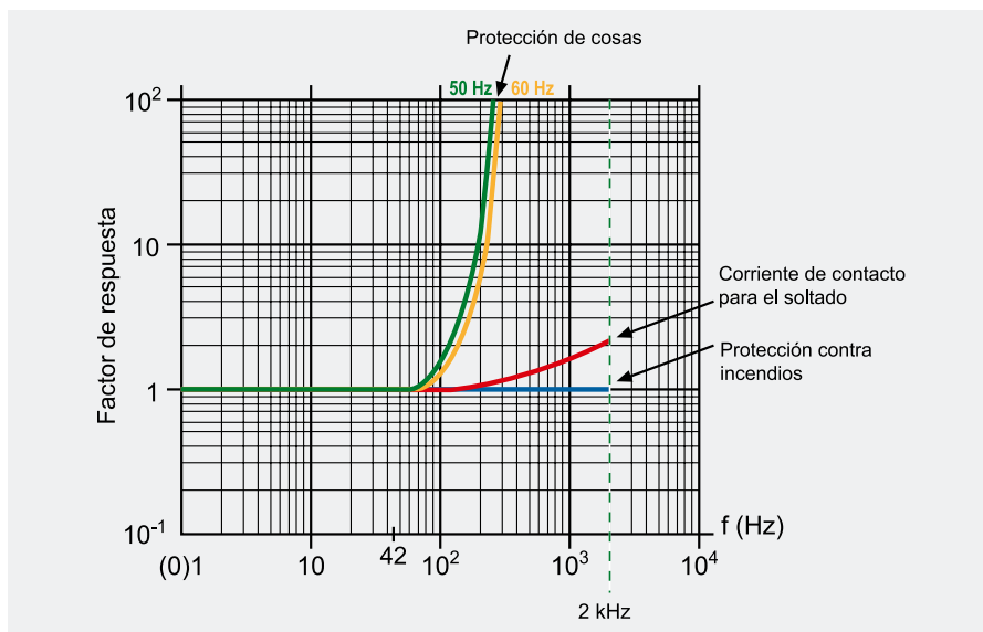
Respuesta en frecuencia según los objetivos de protección
