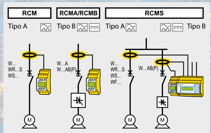
Aplicación de RCM/RCMA/RCMB/RCMS
