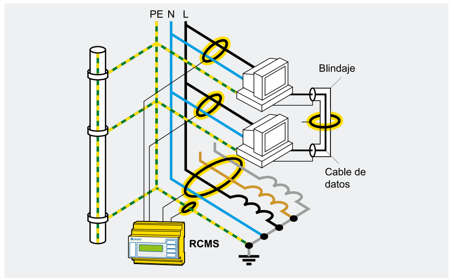
Sistema TN-S ventajoso para la compatibilidad electromagnética (5 conductores) en instalaciones informáticas
