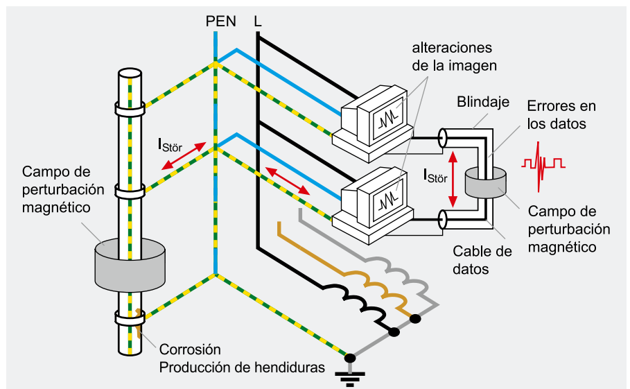
Sistema TN-C no favorable para la compatibilidad electromagnética (4 conductores)
