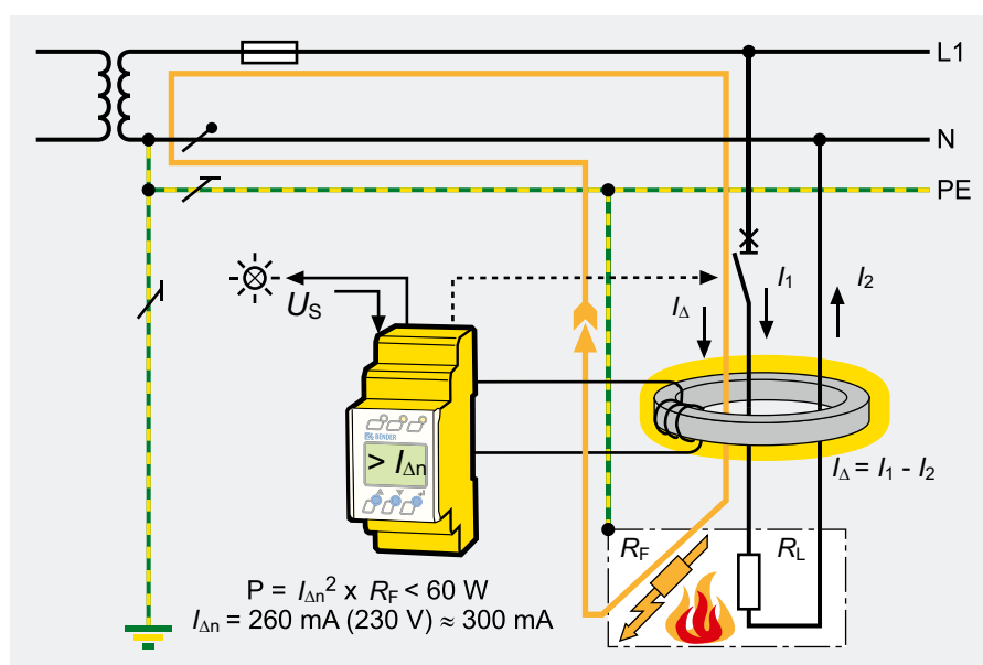
Riesgo de incendio a causa de fallos de aislamiento (a partir de 60 W)
