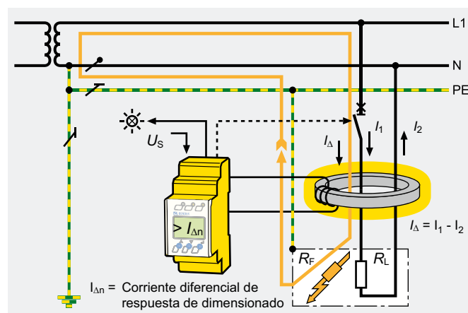
Principio de funcionamiento de un RCM tipo A
